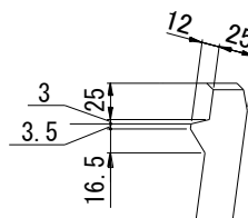
手掛け部詳細図
