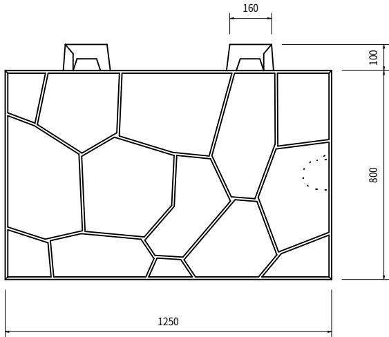
正面断面図
