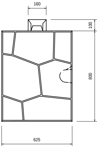
正面断面図
