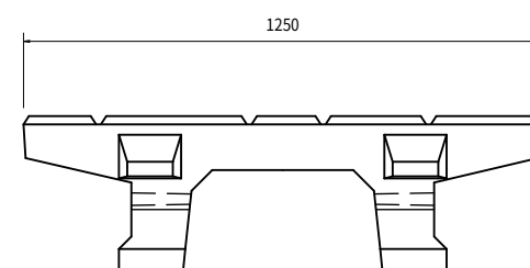
下面断面図
