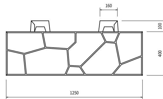
正面断面図
