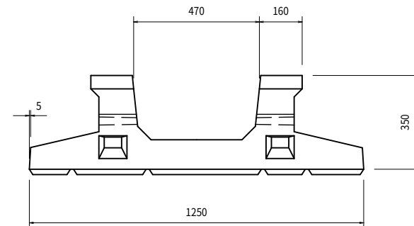
上面断面図
