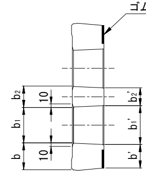
A-A'断面
