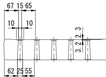
B-B'断面
