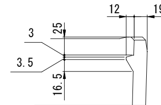
手掛け部詳細図
