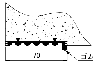
ゴム部詳細図
