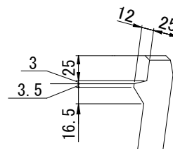
手掛け部詳細図
