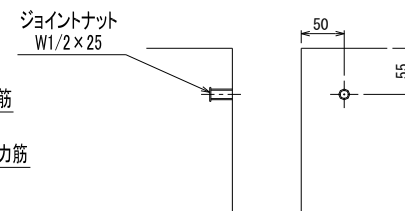
ジョイント部詳細図
