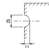
目地部詳細図
