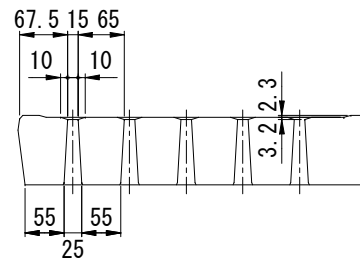
B-B' 断面
