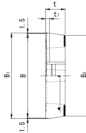
B-B' 断面
