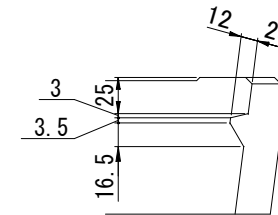
手掛け部詳細図
