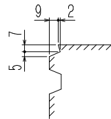
外目地詳細図
