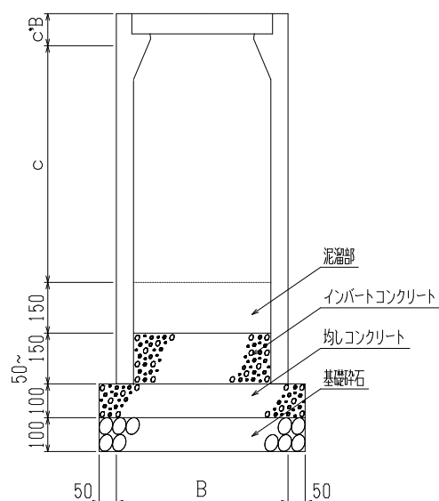
標準断面図
