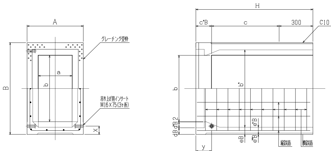
標準断面図
